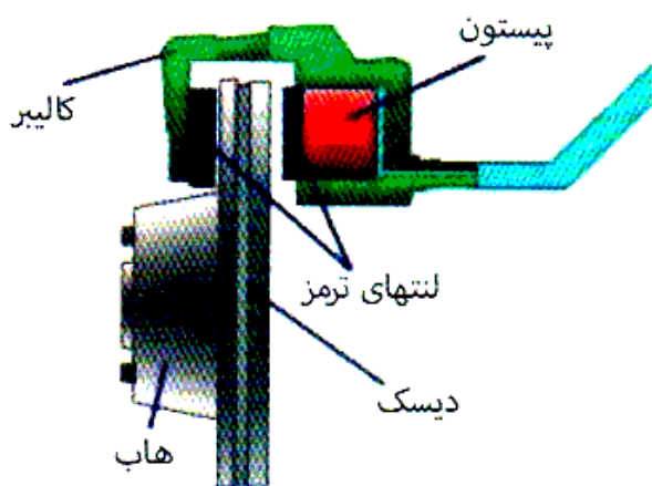
شماتیک ترمز دیسکی
