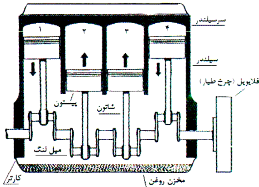
نمایی از موتور و قسمت‌هایی داخل آن
