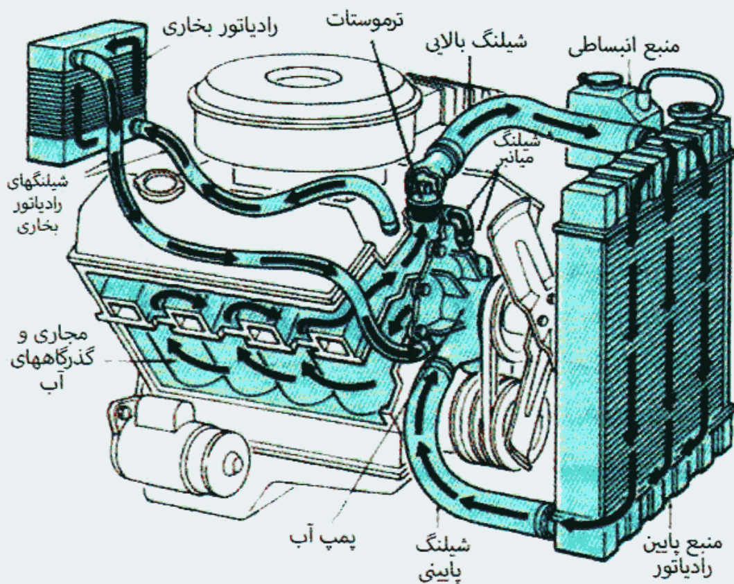
یک نوع سیستم خنک کاری
