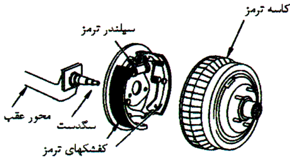
نمونه باز شده ترمز کاسه ای
